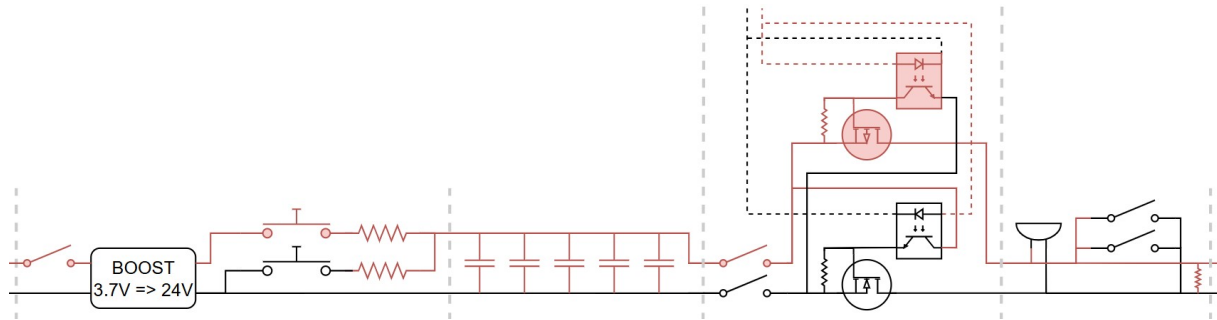
FIGURE 1.7 – Schéma de la ligne de mise à feu
