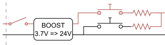
FIGURE 1.8 – Zoom sur le circuit de charge/décharge des condensateurs
