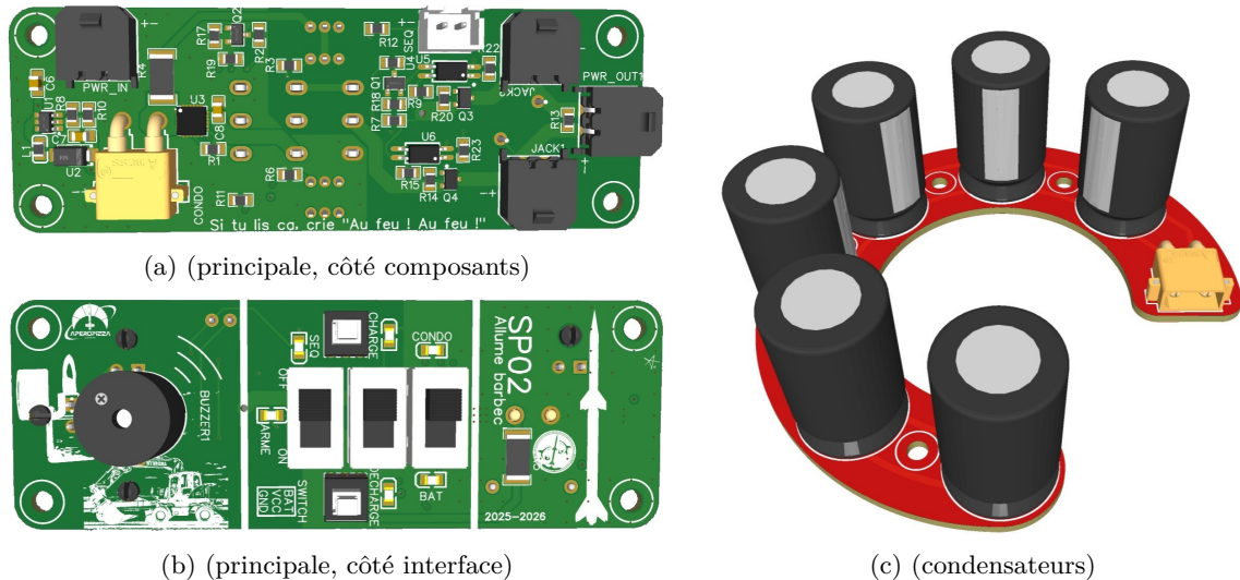
FIGURE 1.5 – Rendu 3D des cartes PCBs principale et condensateurs dy système d'allumage
