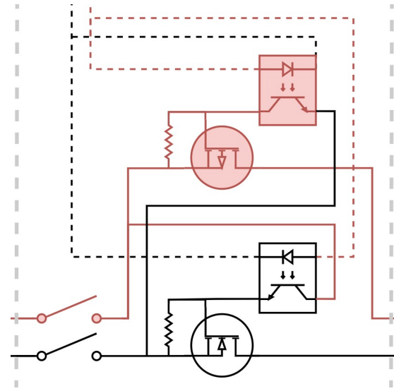
FIGURE 1.10 – Zoom sur le circuit isolateur
